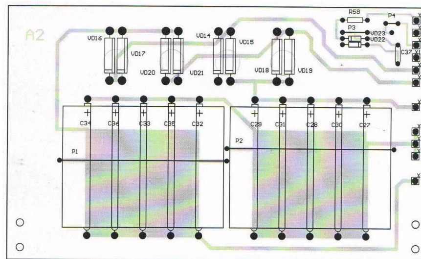
Приложение №3. Печатная плата источника питания - A2
