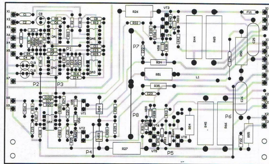
Приложение №2. Печатная плата усилителя - A1
