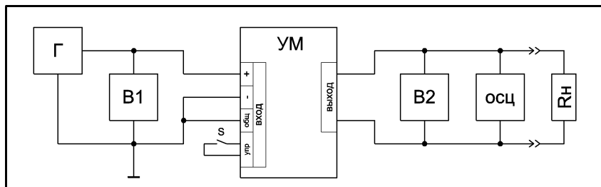
Рис.2 Схема измерений
