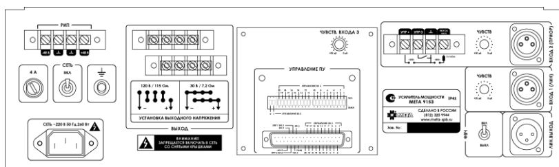
Задняя панель
